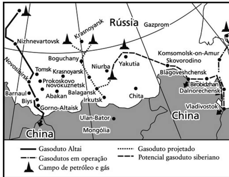
Figura 24.4 — Gasodutos russos na fronteira com a China Fonte: Gazprom
